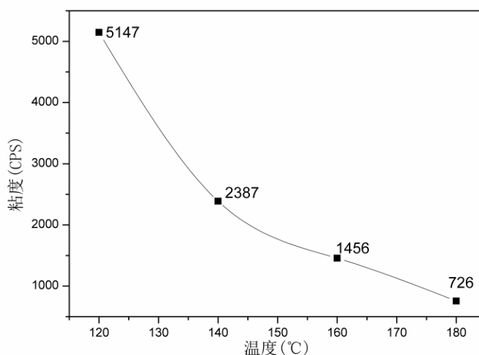
图1、热熔胶粘度随温度变化曲线
